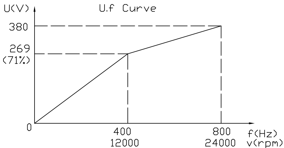
频压曲线
