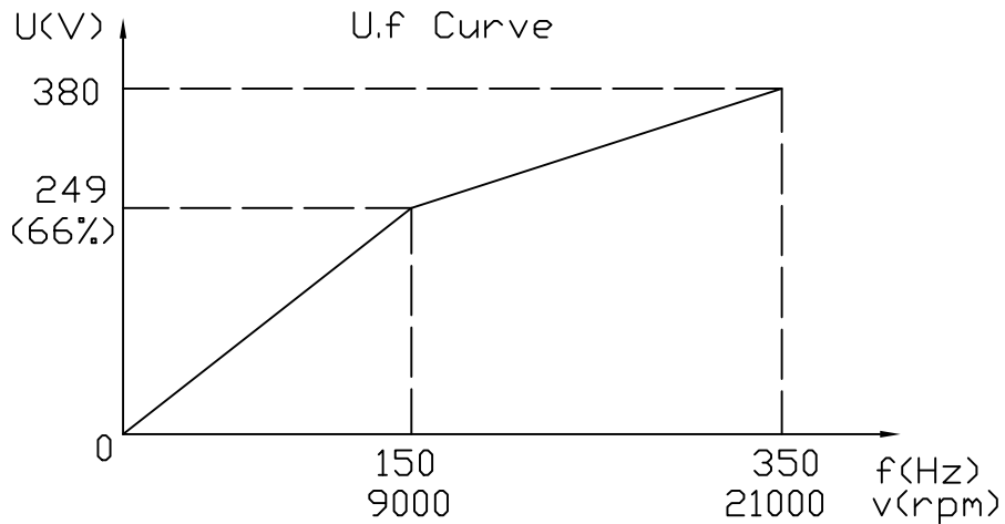
频压曲线
