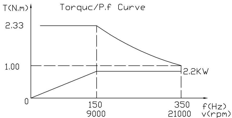
扭矩/功率曲线
